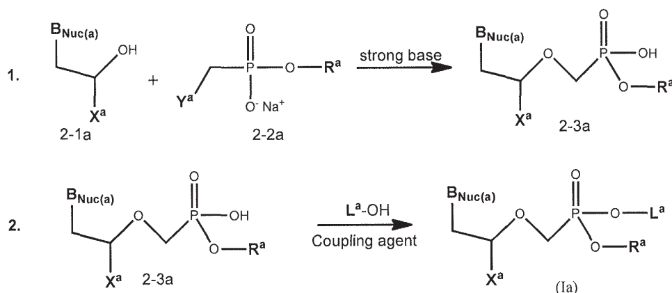
Scheme 2a
