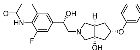
(1S,3aS,5S,6aR)-isomer
