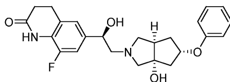
(1R,3aS,5S,6aR)-isomer
