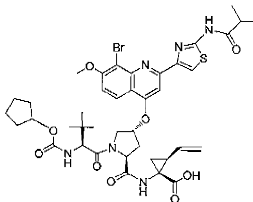
BI-201335
