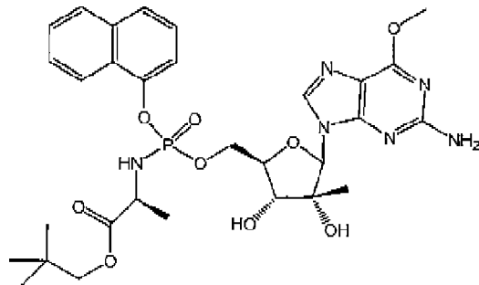
INX-189
