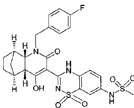
ANA-598 (Setrobuvir)
