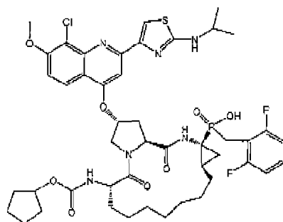
GS-9256
