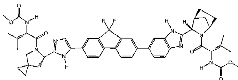
GS-5885
