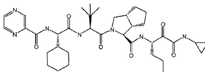
Telaprevir
