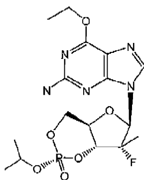
PSI-352938
