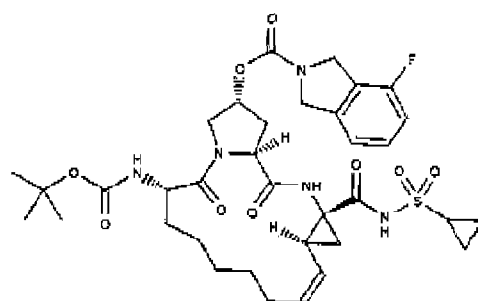
danoprevir
