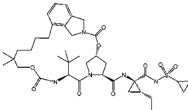
Vaniprevir, MK-7009
