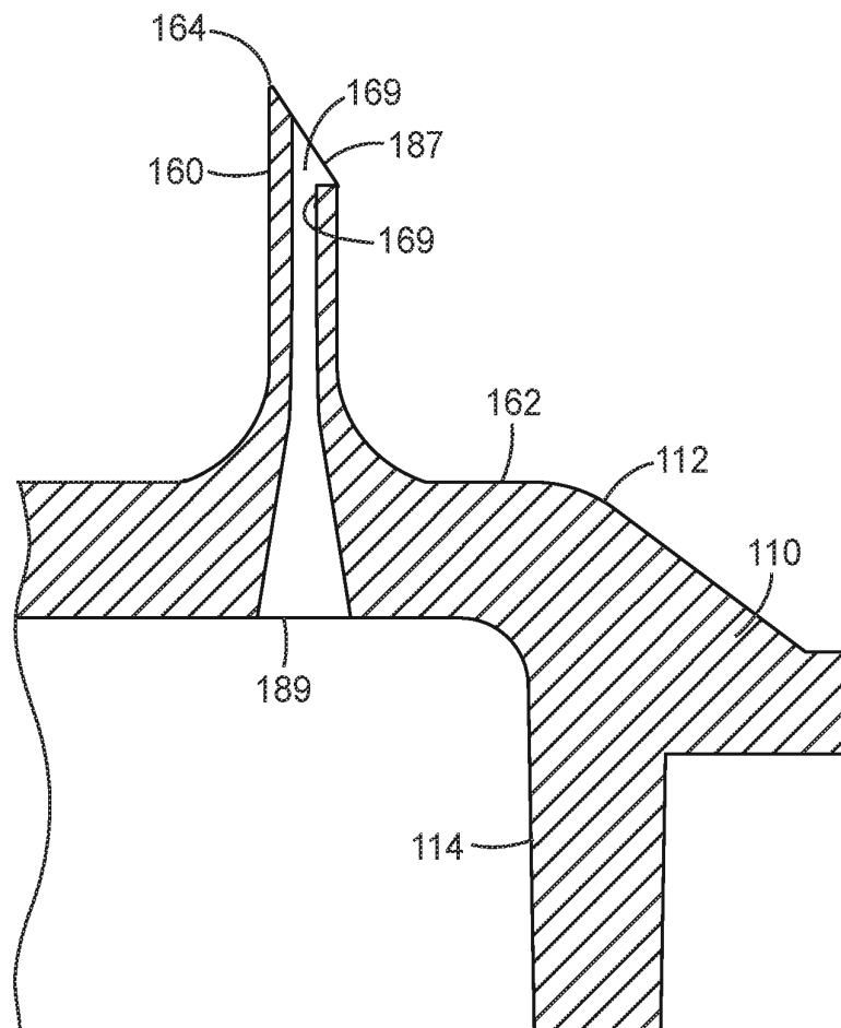
FIG. 4A
