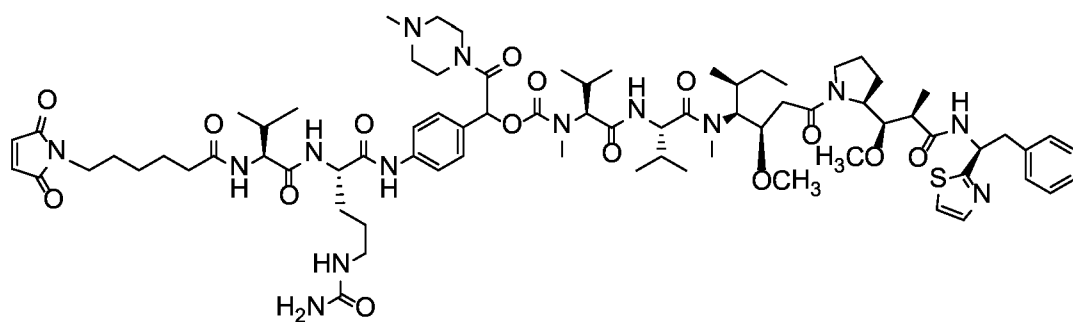
(XI)
