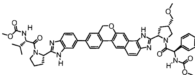
methyl ((2S)-2-(((2S,4S)-2-(9-(2-((2S)-1-((2S)-2-((methoxycarbonyl)amino)-3-methylbutanoyl)pyrrolidin-2-yl)-1H-benzo[d]imidazol-6-yl)-1,11-dihydroisochromeno[4',3':6,7]naphtho[1,2-d]imidazol-2-yl)-4-(methoxymethyl)pyrrolidin-1-yl)-2-oxo-1-phenylethyl)carbamate
