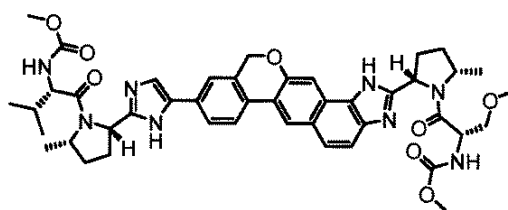
methyl [(2S)-1-((2S,5S)-2-[5-(2-((2S,5S)-1-[N-(methoxycarbonyl)-O-methyl-L-seryl]-5-methylpyrrolidin-2-yl)-1,11-dihydroisochromeno[4',3':6,7]naphtho[1,2-d]imidazol-9-yl)-1H-imidazol-2-yl]-5-methylpyrrolidin-1-yl)-3-methyl-1-oxobutan-2-yl]carbamate
