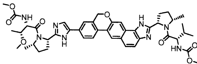
methyl ((2S)-1-((2S,4S)-2-(5-(2-((2S,5S)-1-((2S,3R)-3-methoxy-2-((methoxycarbonyl)amino)butanoyl)-5-methylpyrrolidin-2-yl)-1,11-dihydroisochromeno[4',3':6,7]naphtho[1,2-d]imidazol-9-yl)-1H-imidazol-2-yl)-5-methylpyrrolidin-1-yl)-3-methyl-1-oxobutan-2-yl)carbamate
