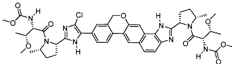
methyl [(2S,3R)-1-((2S,5S)-2-[9-(4-chloro-2-((2S,5S)-1-[N-(methoxycarbonyl)-O-methyl-L-threonyl]-5-methylpyrrolidin-2-yl)-1H-imidazol-5-yl)-1,11-dihydroisochromeno[4',3':6,7]naphtho[1,2-d]imidazol-2-yl]-5-methylpyrrolidin-1-yl)-3-methoxy-1-oxobutan-2-yl]carbamate
