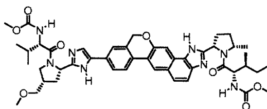
methyl {(2S,3S)-1-[(2S,5S)-2-(9-{2-[(2S,4S)-1-[(2S)-2-[(methoxycarbonyl)amino]-3-methylbutanoyl]-4-(methoxymethyl)pyrrolidin-2-yl]-1H-imidazol-5-yl)-1,11-dihydroisochromeno[4',3':6,7]naphtho[1,2-d]imidazol-2-yl)-5-methylpyrrolidin-1-yl]-3-methyl-1-oxopentan-2-yl]carbamate
