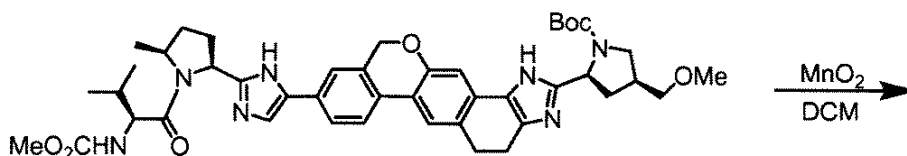
tert-butyl (2S,4S)-2-[9-(2-((2S,5S)-1-[N-(methoxycarbonyl)-L-valyl]-5-methylpyrrolidin-2-yl)-1H-imidazol-5-yl)-1,4,5,11-tetrahydroisochromeno[4',3':6,7]naphtho[1,2-d]imidazol-2-yl)-4-(methoxymethyl)pyrrolidine-1-carboxylate
