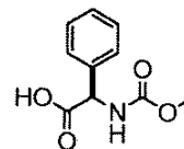
(R)-2-(methoxycarbonylamino)-2-phenylacetic acid
