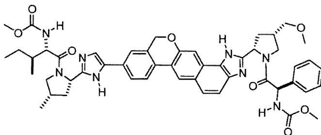
methyl ((1R)-2-((2S,4S)-2-[9-(2-((2S,4S)-1-((2S,3R)-2-((methoxycarbonyl)amino)-3-methylpentanoyl)-4-methylpyrrolidin-2-yl)-1H-imidazol-5-yl)-1,11-dihydroisochromeno[4',3':6,7]naphtho[1,2-d]imidazol-2-yl)-4-(methoxymethyl)pyrrolidin-1-yl]-2-oxo-1-phenylethyl)carbamate
