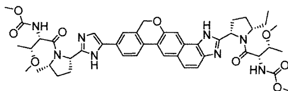
methyl[(2S,3R)-1-((2S,5S)-2-[5-(2-((2S,5S)-5-ethyl-1-[N-(methoxycarbonyl)-O-methyl-L-threonyl]pyrrolidin-2-yl)-1,11-dihydroisochromeno[4',3':6,7]naphtho[1,2-d]imidazol-9-yl)-1H-imidazol-2-yl]-5-methylpyrrolidin-1-yl)-3-methoxy-1-oxobutan-2-yl]carbamate
