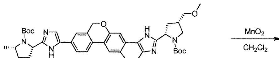
tert-butyl (2S,5S)-2-(9-((2S,5S)-1-(tert-butoxycarbonyl)-4-(methoxymethyl)pyrrolidin-2-yl)-1H-imidazol-5-yl)-1,4,5,11-tetrahydroisochromeno[4',3':6,7]naphtho[1,2-d]imidazol-2-yl)-5-methylpyrrolidine-1-carboxylate
