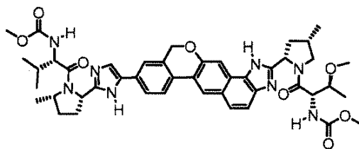
methyl ((2S)-1-((2S,5S)-2-(5-{2-[(2S,4S)-1-((2S,3S)-3-methoxy-2-[(methoxycarbonyl)amino]butanoyl}-4-methylpyrrolidin-2-yl)-1,11-dihydroisochromeno[4',3':6,7]naphtho[1,2-d]imidazol-9-yl)-1H-imidazol-2-yl)-5-methylpyrrolidin-1-yl]-3-methyl-1-oxobutan-2-yl)carbamate
