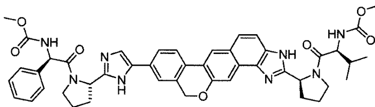
methyl [1-(2-{5-[2-(1-[(methoxycarbonyl)amino]-3-methyl-1-oxobutan-2-yl]pyrrolidin-2-yl)-1,11-dihydroisochromeno[4',3':6,7]naphtho[1,2-d]imidazol-9-yl]-1H-imidazol-2-yl]pyrrolidin-1-yl)-phenyl-1-oxoacet-2-yl]carbamate
