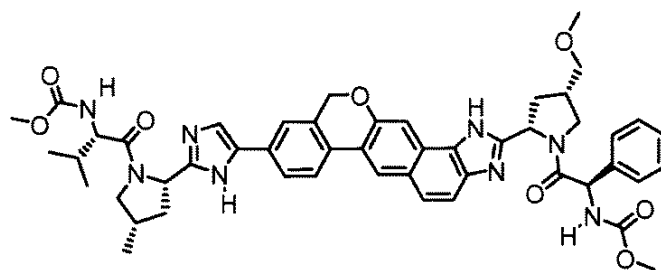
methyl ((2S)-1-[(2S,4S)-2-(5-(2-[(2S,4S)-1-[(2R)-2-[(methoxycarbonyl)amino]-2-phenylacetyl]-4-(methoxymethyl)pyrrolidin-2-yl)-1,11-dihydroisochromeno[4',3':6,7]naphtho[1,2-d]imidazol-9-yl)-1H-imidazol-2-yl)-4-methylpyrrolidin-1-yl]-3-methyl-1-oxobutan-2-yl)carbamate
