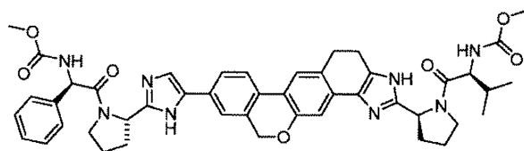
methyl [1-(2-{5-[2-(1-((methoxycarbonyl)amino)-3-methyl-1-oxobutan-2-yl)pyrrolidin-2-yl]-1,4,5,11-tetrahydroisochromeno[4',3':6,7]naphtho[1,2-d]imidazol-9-yl)-1H-imidazol-2-yl}pyrrolidin-1-yl)-phenyl-1-oxoacet-2-yl]carbamate
