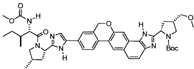
tert-butyl (2S,4S)-2-[9-(2-((2S,4S)-1-[N-(methoxycarbonyl)-L-alloisoleucyl]-4-methylpyrrolidin-2-yl)-1H-imidazol-5-yl)-1,11-dihydroisochromeno[4',3':6,7]naphtho[1,2-d]imidazol-2-yl]-4-(methoxymethyl)pyrrolidine-1-carboxylate
