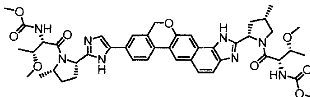
methyl [(2S,3R)-3-methoxy-1-[(2S,5S)-2-[9-(2-{(2S,5S)-1-[N-(methoxycarbonyl)-O-methyl-L-threonyl]-5-methylpyrrolidin-2-yl]-1H-imidazol-5-yl)-1,11-dihydroisochromeno[4',3':6,7]naphtho[1,2-d]imidazol-2-yl]-4-methylpyrrolidin-1-yl]-1-oxobutan-2-yl]carbamate
