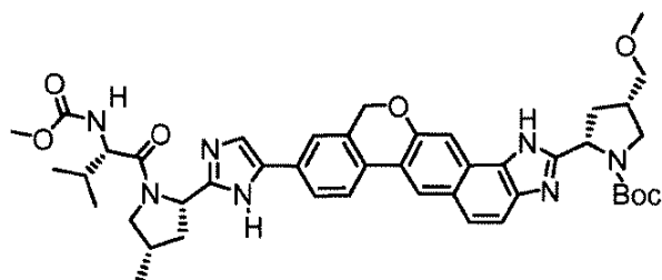
tert-butyl (2S,4S)-2-[9-(2-((2S,4S)-1-[N-(methoxycarbonyl)-L-valyl]-4-methylpyrrolidin-2-yl)-1H-imidazol-5-yl)-3,11-dihydroisochromeno[4',3':6,7]naphtho[1,2-d]imidazol-2-yl]-4-(methoxymethyl)pyrrolidine-1-carboxylate
