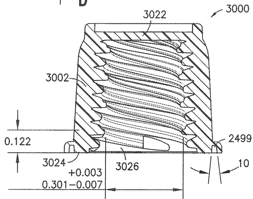
SECTION AC-AC FIG. 24E
