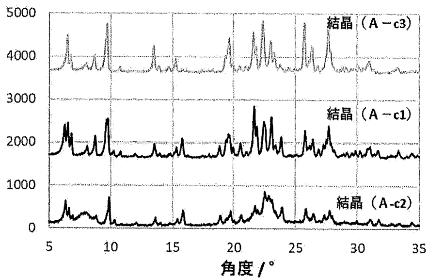
実施例、比較例の結晶 (A) のXRDチャート
