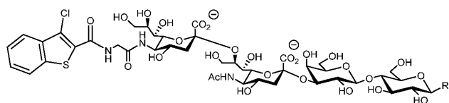
[00942] Compound D112
