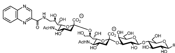
[00963] Compound D217
