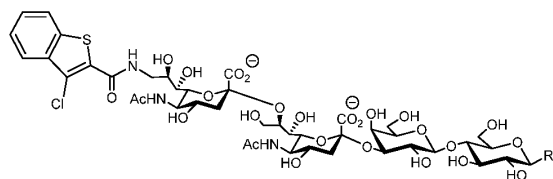
[00959] Compound D213
