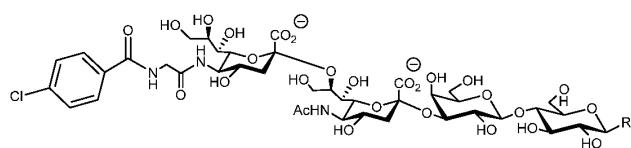
[00939] Compound D109
