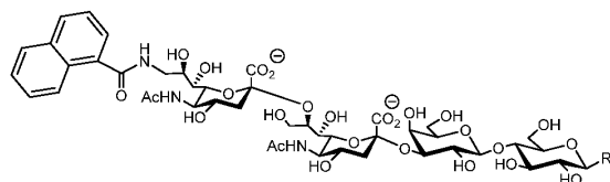
[00949] Compound D203
