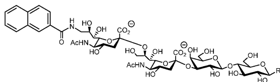
[00948] Compound D202
