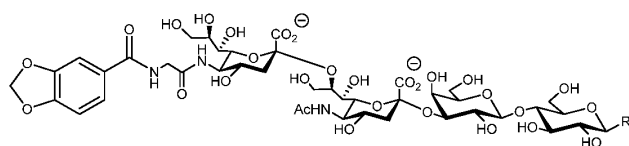
[00945] Compound D116
