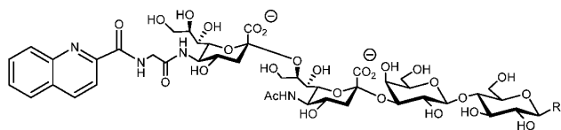
[00937] Compound D107
