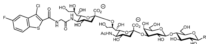
[00942] Compound D112
