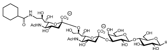
[00961] Compound D215
