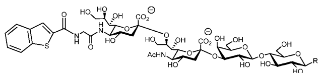
[00941] Compound D111
