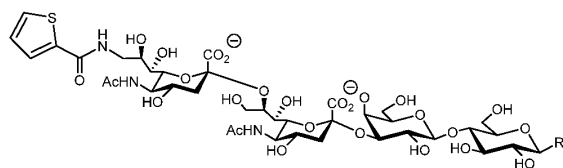
[00950] Compound D204
