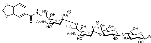
[00962] Compound D216
