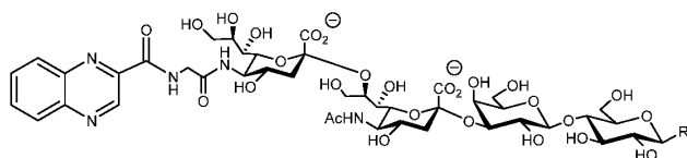
[00946] Compound D117
