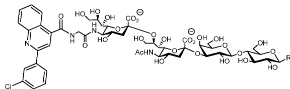
[00947] Compound D201
