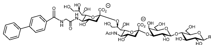
[00938] Compound D108
