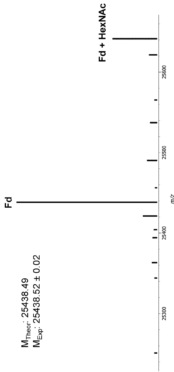
FIG. 2C (Subunit / IdeS)
