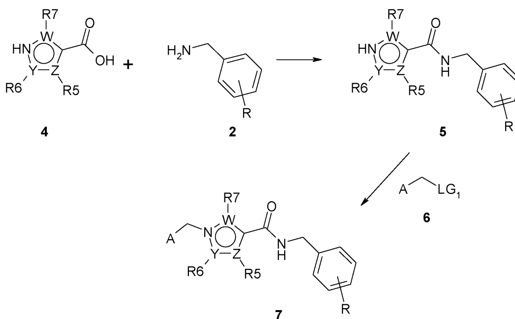
Scheme 2a
