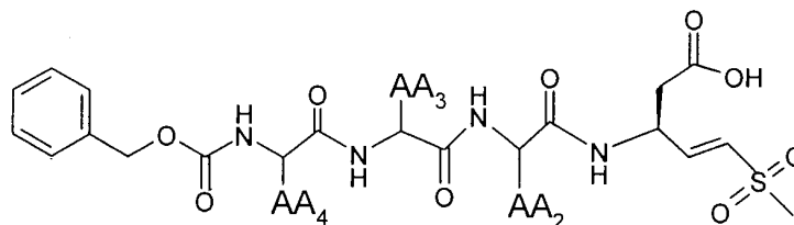
Formula 1e
