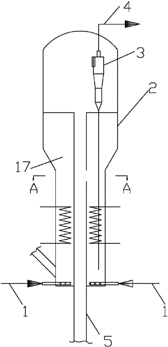
A-A剖面
