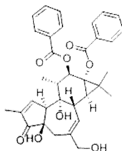
Phorbol 12,13- Dibenzoate
