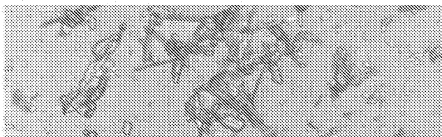
氯化钠水溶液复溶
