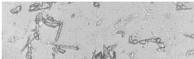
氯化镁水溶液复溶
