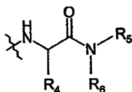
(IIA)
