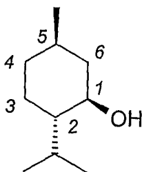
(-)-menthol
