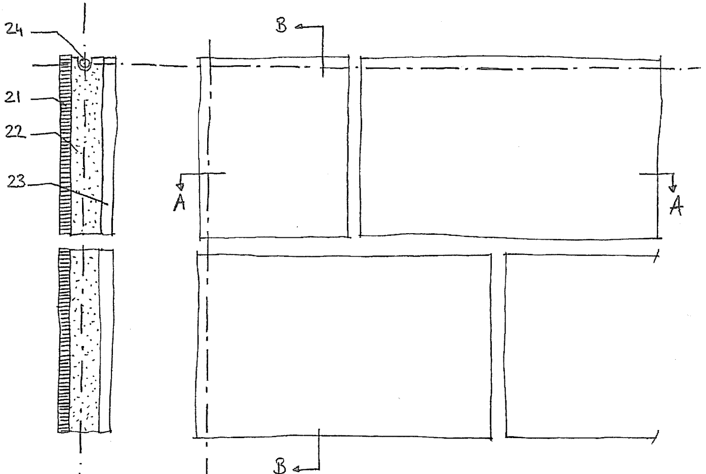
COUPE B-B Fig. 3D
