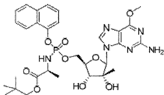
INX-189
