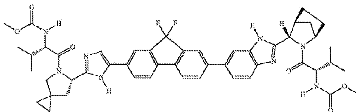
GS-5885
