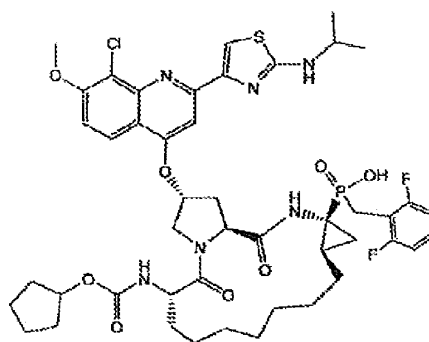
GS-9256
