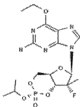
PSI-352938
