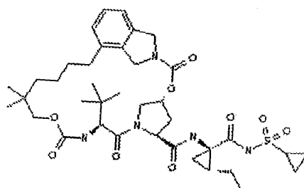
Vaniprevir, MK-7009
