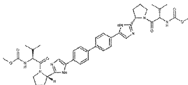
BMS-790052 (daclatasvir)
