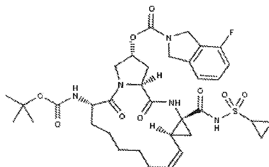
danoprevir
