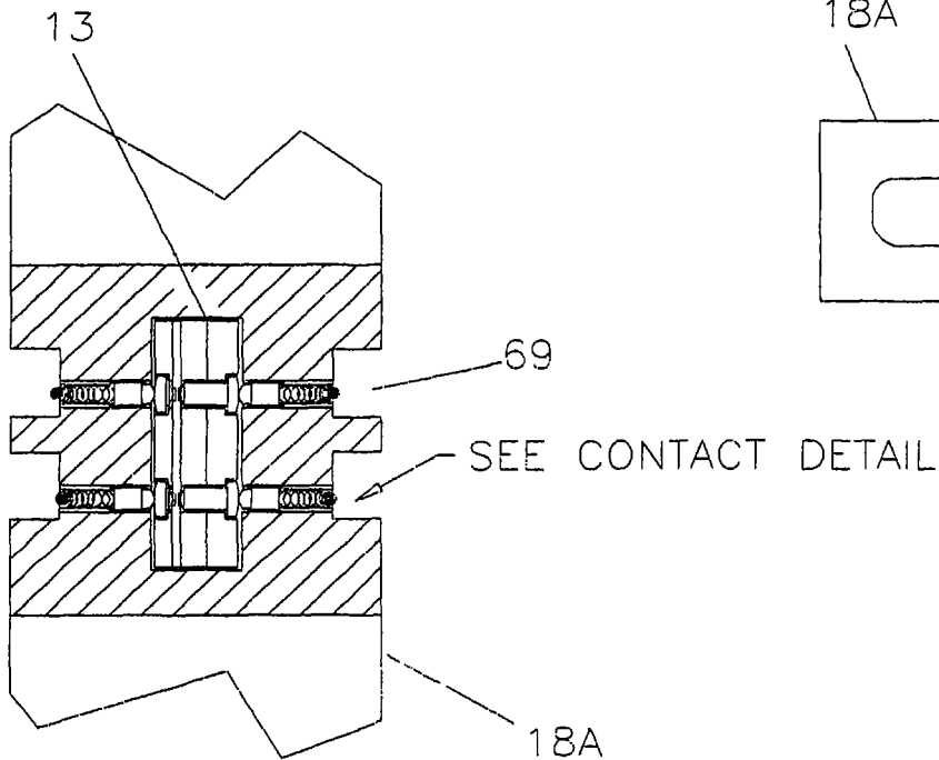
SECTION D-D FIG. 13
