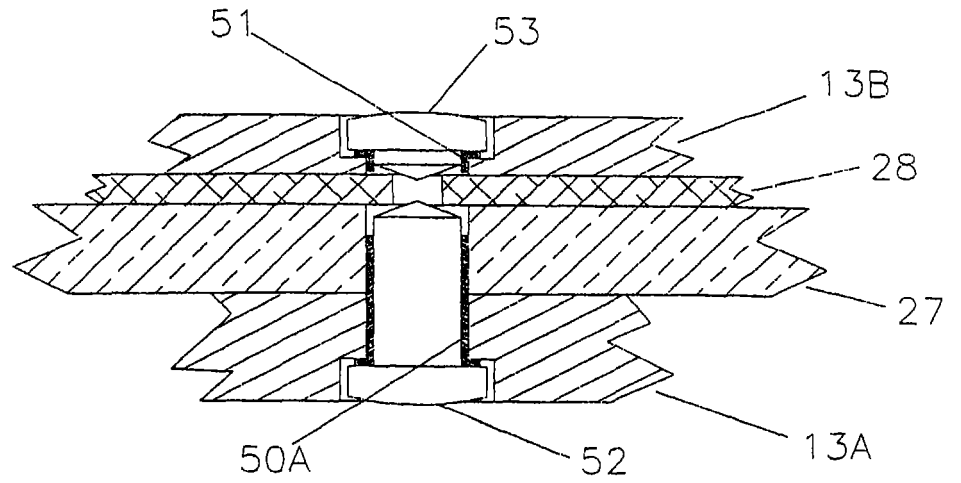
SECTION A-A FIG. 12
