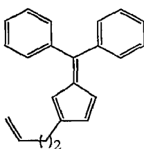
2-(but-3-enyl)-6,6-diphenylpentafulvene
