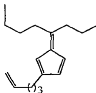
2-(pent-4-enyl)-6,6-dibutylpentafulvene
