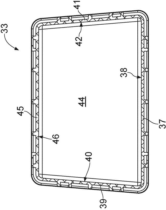
A-A FIG. 8
