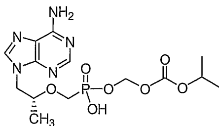
mono-POC PMPA
