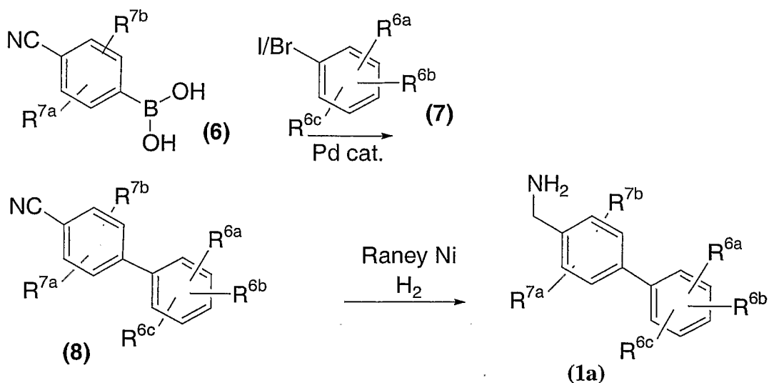
SCHEME 2a
