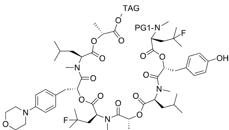
(II-9)
