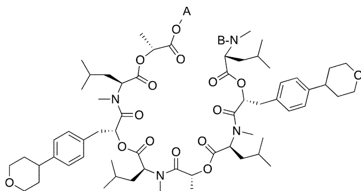
(II-5a)
