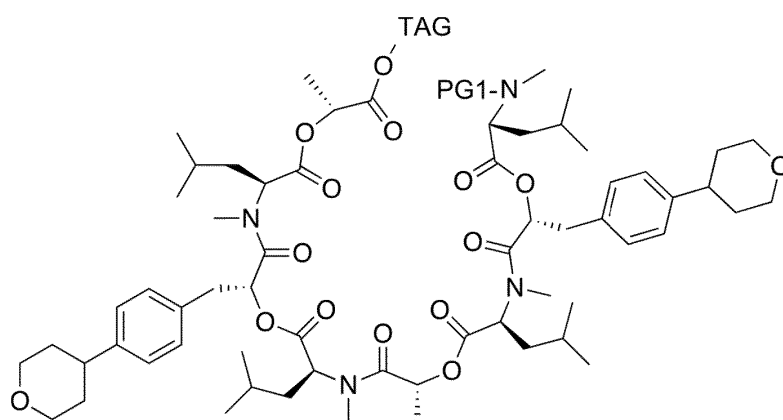
(II-4b)
