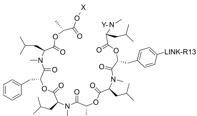
(II-12b)
