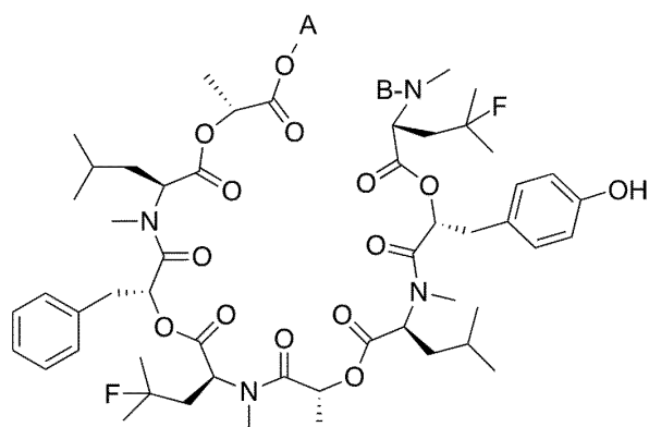
(II-10a)
