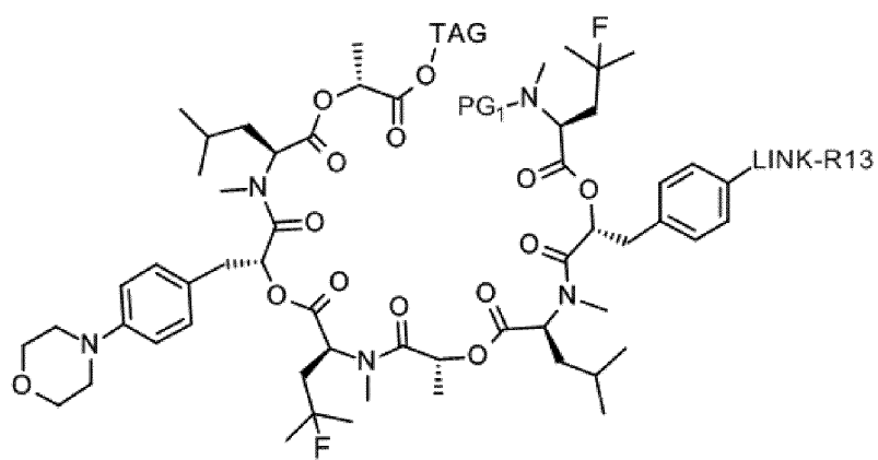
(II-12b)
