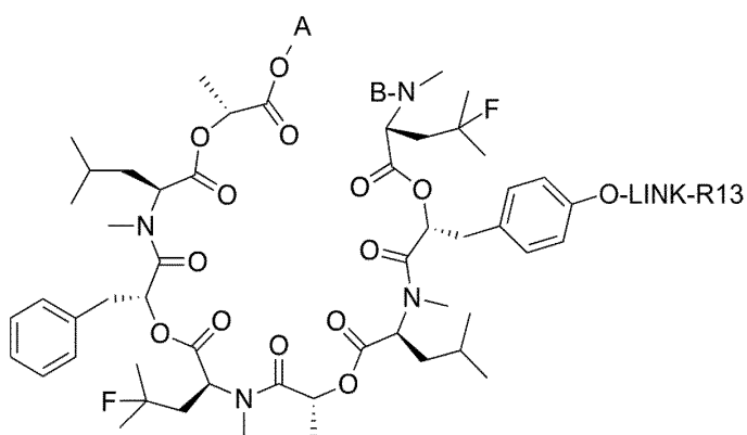
(II-14a)
