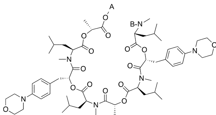
(II- 1a)
