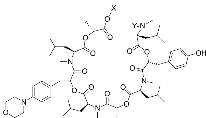
(II-7b)
