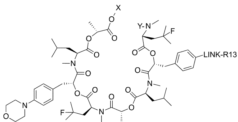
(II-13b)
