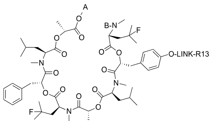
(II-14a)
