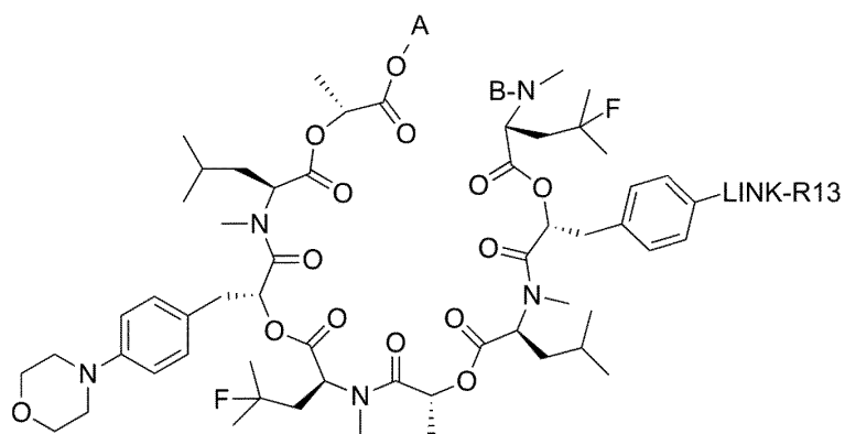
(II-13a)
