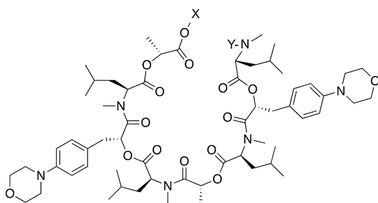
(II- 1b)
