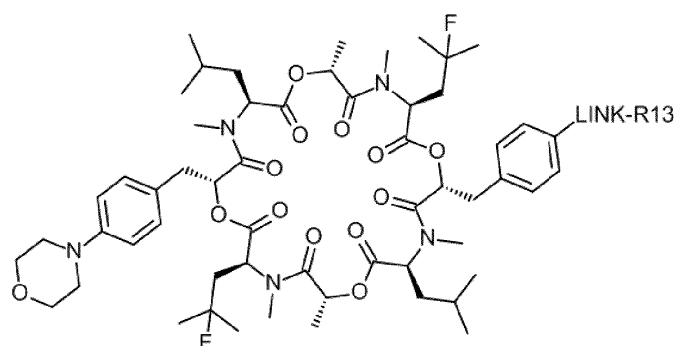
(I-4)
