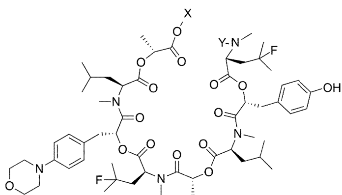
(II-9b)
