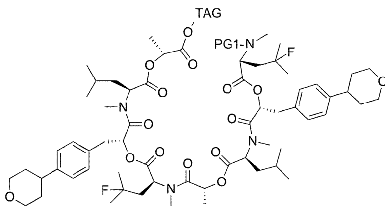
(II-6)
