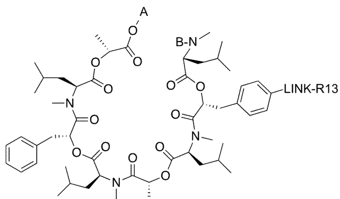
(II-12a)
