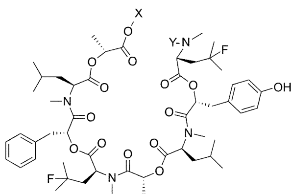
(II-10b)
