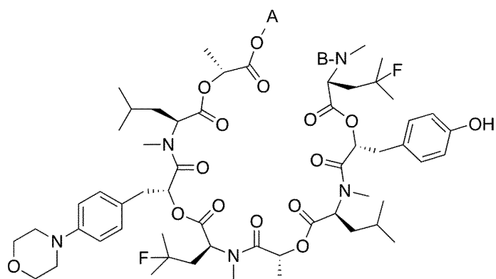
(II-9a)
