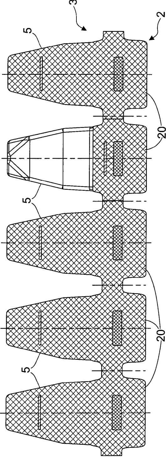
Fig. 5 (A-A)
