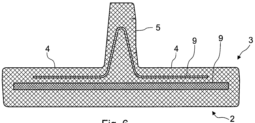
Fig. 6 (D-D)
