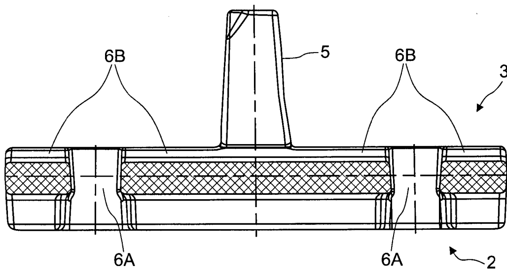
Fig. 7 (E-E)
