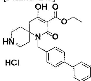
[Formula 243]
