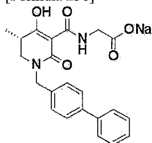
[Formula 236]
