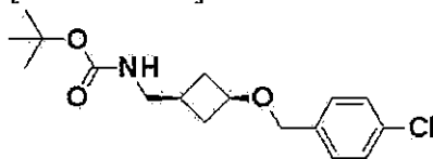
[Formula 171]
