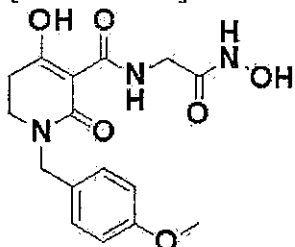
[Formula 250]
