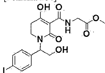
[Formula 264]
