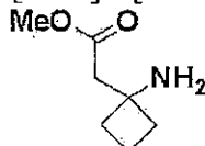
[0176] [Formula 25]
