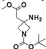
[Formula 23]
