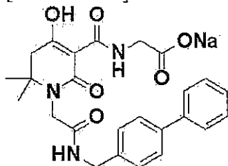
[Formula 256]
