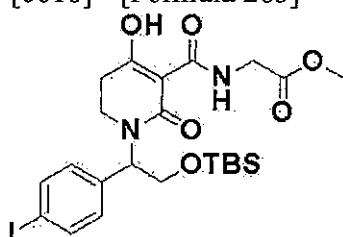
[0618] [Formula 263]
