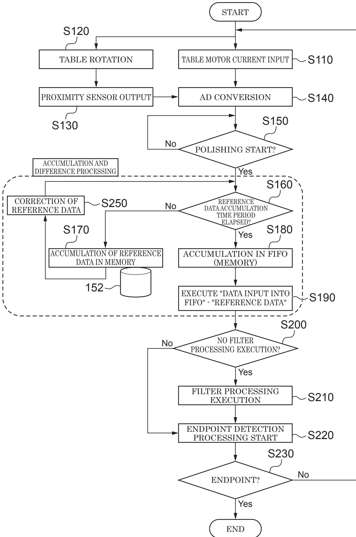
FIG. 23
