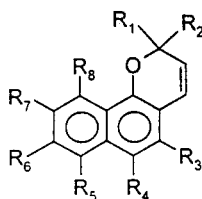
2H-Naphthopyrans
