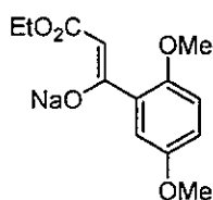
Sodium 1-(2,5-dimethoxyphenyl)-3-ethoxy-3-oxoprop-1-en-1-olate
