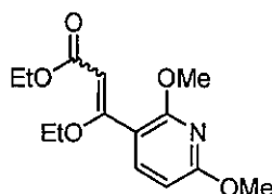
(Z,E)-Ethyl 3-(2,6-dimethoxypyridin-3-yl)-3-ethoxyacrylate
