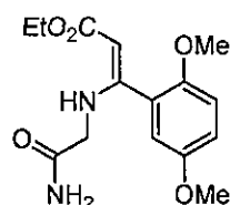
(Z)-Ethyl 3-((2-amino-2-oxoethyl)amino)-3-(2,5-dimethoxyphenyl)acrylate
