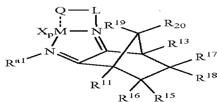
Structure 19e
