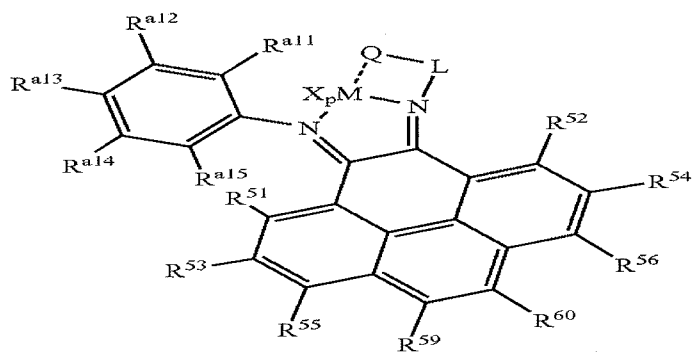
Structure 39e
