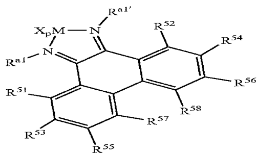
Structure 12e
