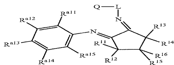
Structure 30f
