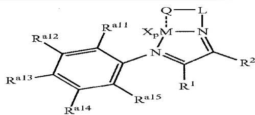
Structure 27e
