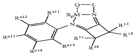
Structure 29e
