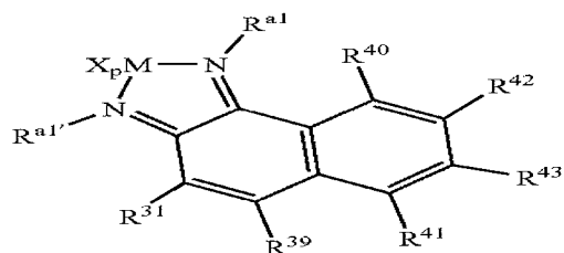
Structure 10e
