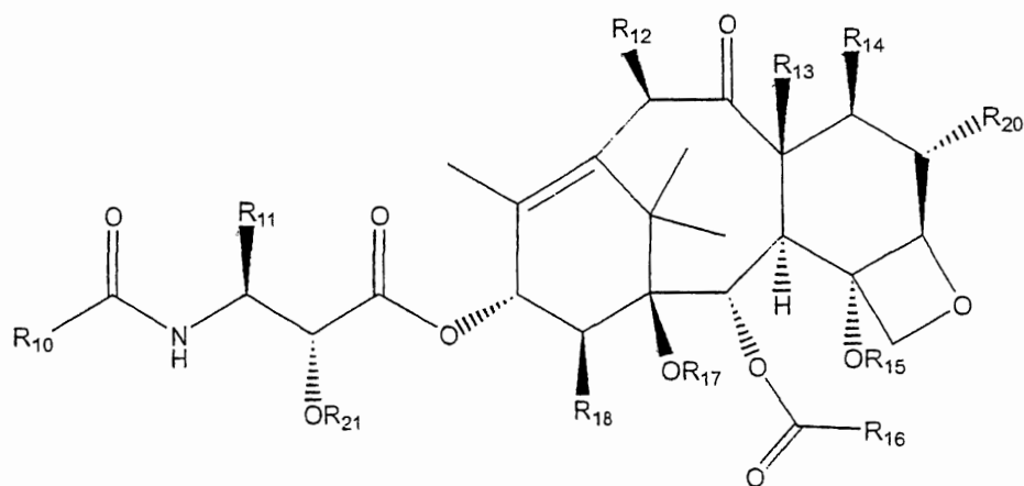
(VII).
