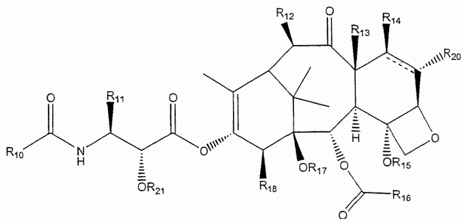
(VIII).
