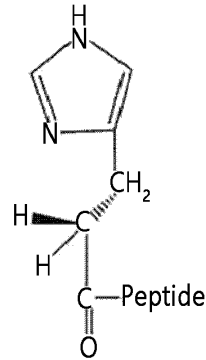
Des-amino-histidyl (DA)-GLP-2
