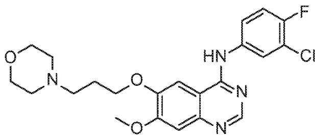
Gefitinib
