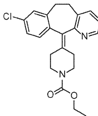
Loratadine
