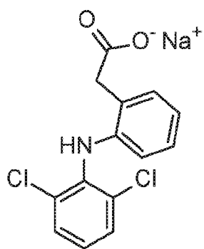
Diclofenac
