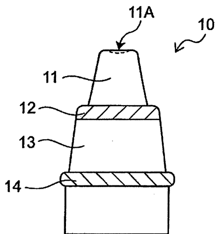
(B)側面図
