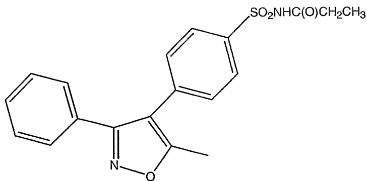
1a
