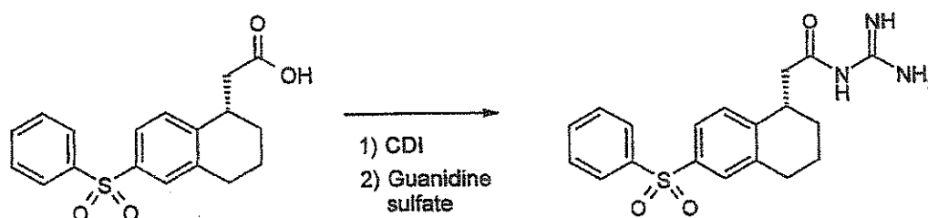
SCHEME Y
