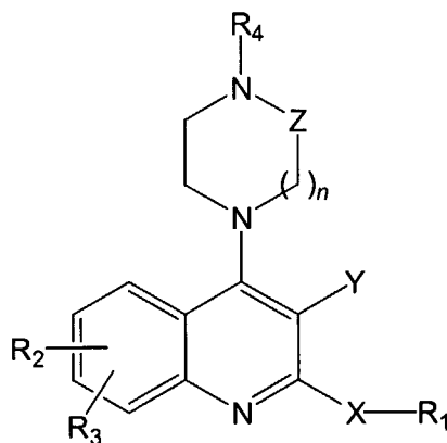
(1b)
