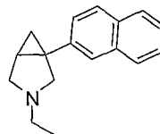
3-ethyl-1-(naphthalen-2-yl)-3-aza- bicyclo[3.1.0]hexane
