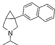
3-isopropyl-1-(naphthalen-2-yl)-3-aza- bicyclo[3.1.0]hexane
