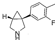
1-(3-fluoro-4-methylphenyl)-3-aza-bicyclo[3.1.0]hexane
