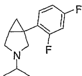
1-(2,4-difluorophenyl)-3-isopropyl-3-aza-bicyclo[3.1.0]hexane
