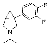
1-(3,4-difluorophenyl)-3-isopropyl-3-aza-bicyclo[3.1.0]hexane
