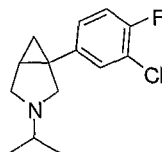
1-(3-chloro-4-fluorophenyl)-3-isopropyl-3-aza-bicyclo[3.1.0]hexane
