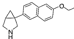
1-(2-ethoxynaphthalen-6-yl)-3-aza- bicyclo[3.1.0]hexane
