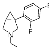
3-ethyl-1-(2,4-difluorophenyl)-3-aza-bicyclo[3.1.0]hexane
