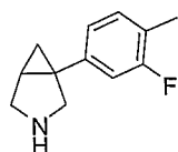
1-(3-fluoro-4-methylphenyl)-3-aza-bicyclo[3.1.0]hexane
