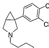
3-butyl-1-(3,4-dichlorophenyl)-3-aza-bicyclo[3.1.0]hexane
