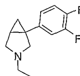
1-(3,4-difluorophenyl)-3-ethyl-3-aza-bicyclo[3.1.0]hexane
