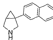
1-(naphthalen-2-yl)-3-aza- bicyclo[3.1.0]hexane
