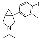
1-(4-fluoro-3-methylphenyl)-3-isopropyl-3-aza-bicyclo[3.1.0]hexane
