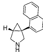
1-(naphthalen-1-yl)-3-aza-bicyclo[3.1.0]hexane
