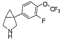
1-(3-fluoro-4-(trifluoromethoxy)phenyl)-3-aza-bicyclo[3.1.0]hexane
