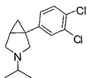
1-(3,4-dichlorophenyl)-3-isopropyl-3-aza-bicyclo[3.1.0]hexane
