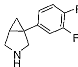
1-(3,4-difluorophenyl)-3-aza-bicyclo[3.1.0]hexane
