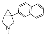
3-methyl-1-(naphthalen-2-yl)-3-aza- bicyclo[3.1.0]hexane
