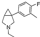
3-ethyl-1-(4-fluoro-3-methylphenyl)-3-aza-bicyclo[3.1.0]hexane
