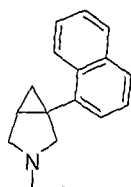
3-methyl-1-(naphthalen-1-yl)-3-aza- bicyclo[3.1.0]hexane
