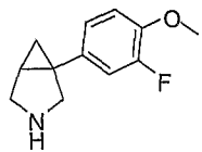
1-(3-fluoro-4-methoxyphenyl)-3-aza-bicyclo[3.1.0]hexane
