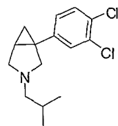
1-(3,4-dichlorophenyl)-3-isobutyl-3-aza-bicyclo[3.1.0]hexane
