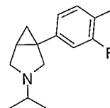
1-(3-fluoro-4-methylphenyl)-3-isopropyl-3-aza-bicyclo[3.1.0]hexane
