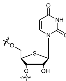
4'Thio-Uridine
