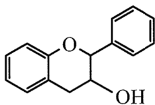
3-flavanol
