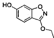
3-ethoxy-benzo[d]isoxazole-6-ol
