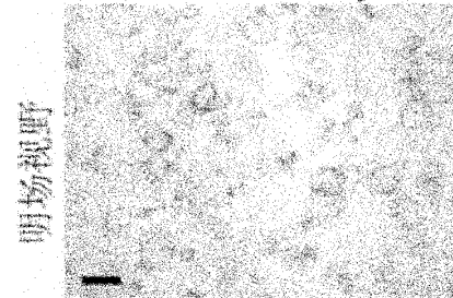
图 39 25-HL 1 \mu\text{M}
