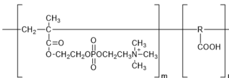
Lipidure® AC 01
