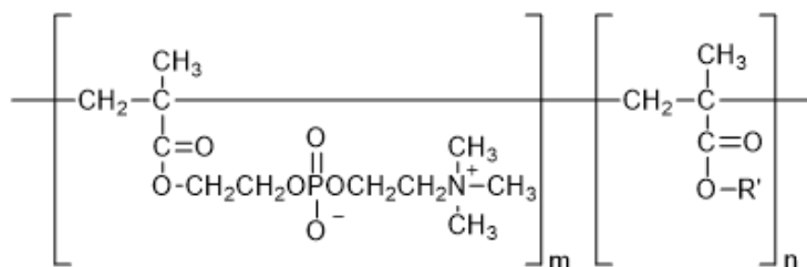
Lipidure® CM5206
