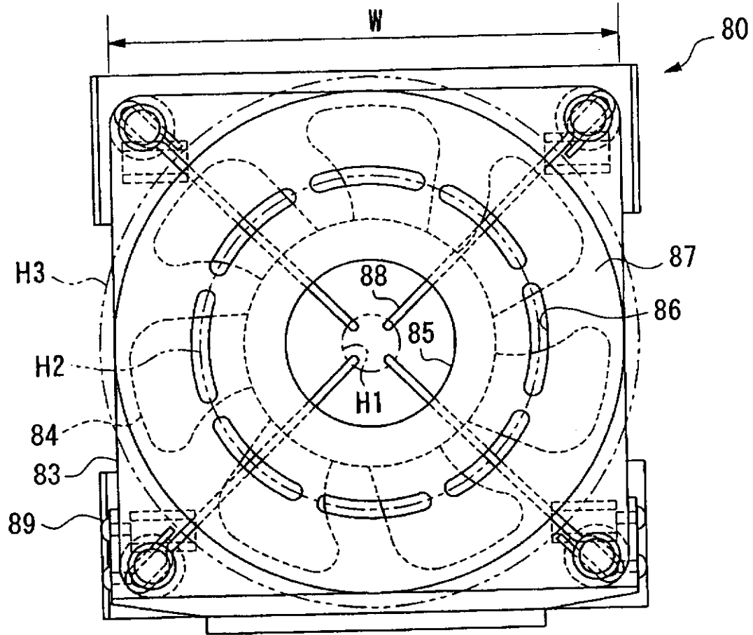
FIG. 7A
