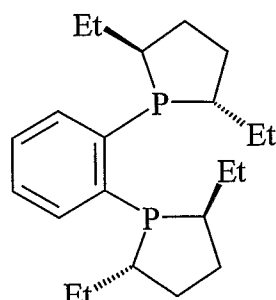
(S,S)-Et-DuPhos,
