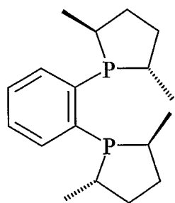
(S,S)-Me-DuPhos
