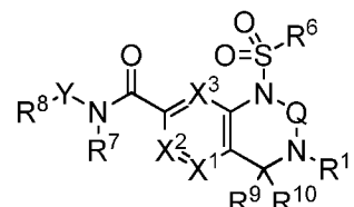
(I-III)
