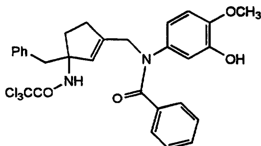
Cpd. 41
