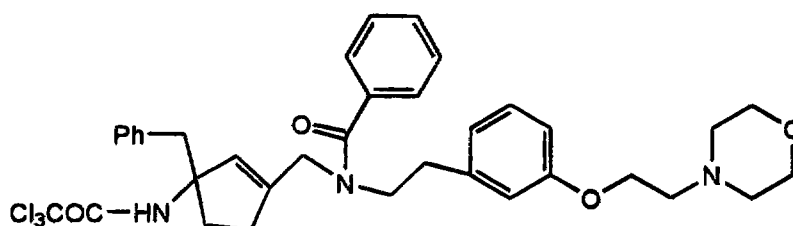
Cpd. 34
