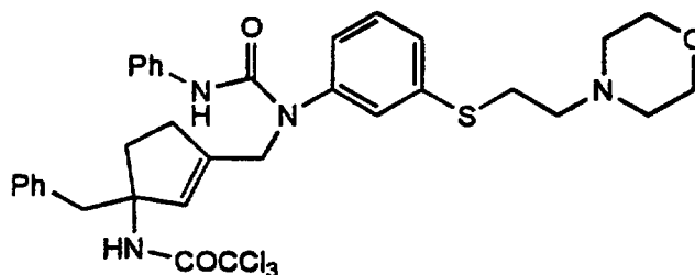
Cpd. 22
