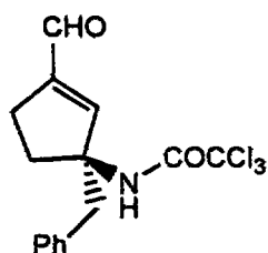
Cpd. 4a
