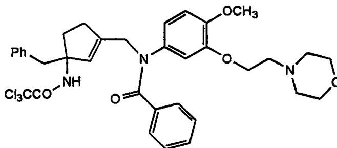
Cpd. 41
