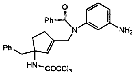
Cpd. 25
