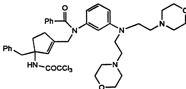
Cpd. 23b
