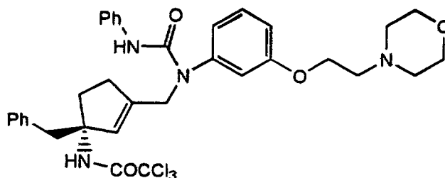
Cpd. 8
