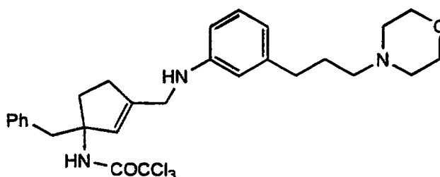
Cpd. 18
