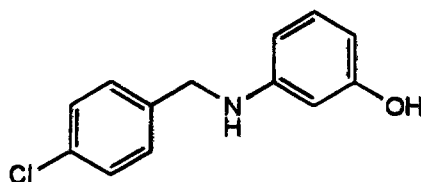
Cpd. 27
