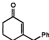
Cpd. 1
