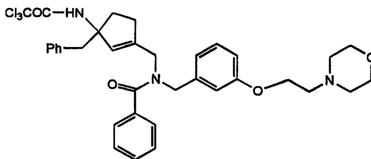
Cpd. 32
