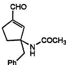
Cpd. 13
