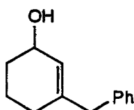
Cpd. 2
