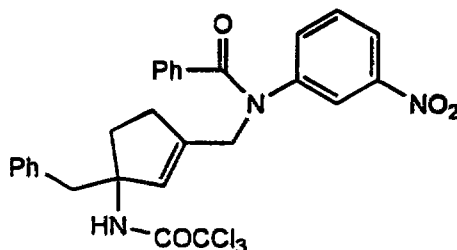
Cpd. 24
