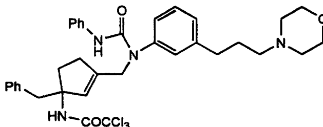
Cpd. 19
