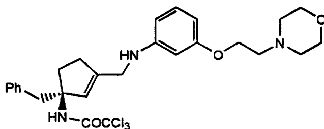
Cpd. 6a
