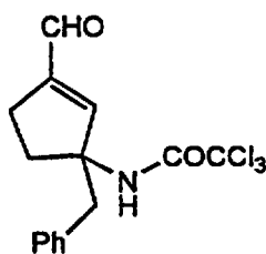
Cpd. 4
