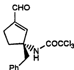
Cpd. 4b
