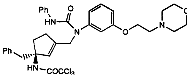
Cpd. 9
