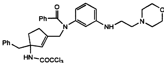
Cpd. 23a
