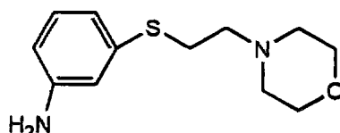
Cpd. 20
