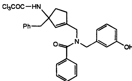
Cpd. 31
