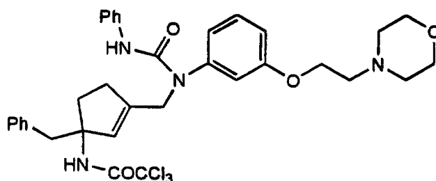
Cpd. 7
