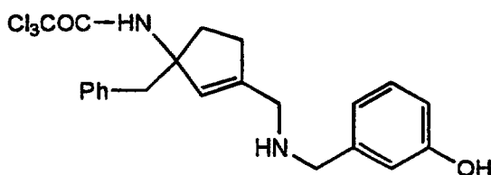
Cpd. 30
