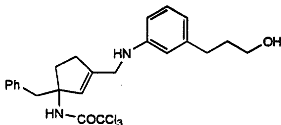
Cpd. 17
