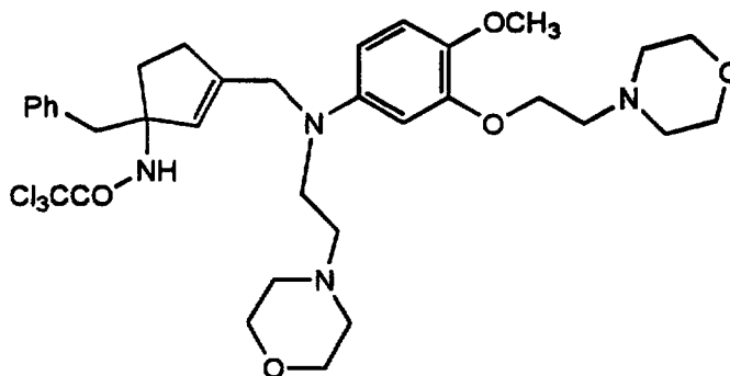
Cpd. 40
