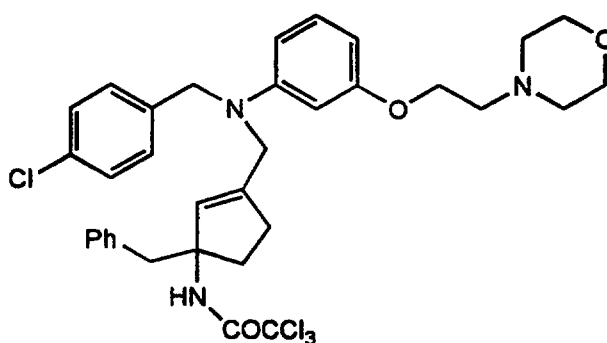
Cpd. 29
