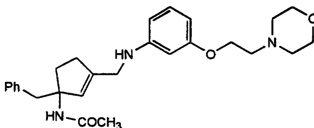
Cpd. 14
