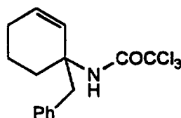
Cpd. 3
