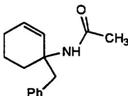
Cpd. 12
