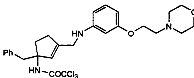
Cpd. 6
