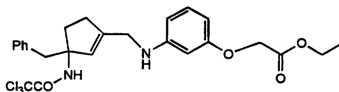
Cpd. 43
