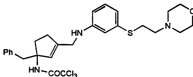
Cpd. 21
