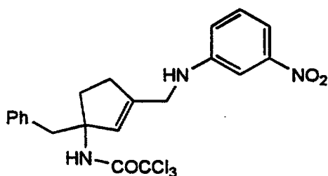
Cpd. 23
