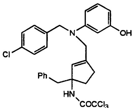
Cpd. 28
