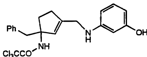
Cpd. 42
