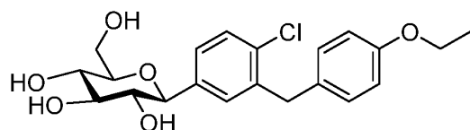
Dapagliflozin
