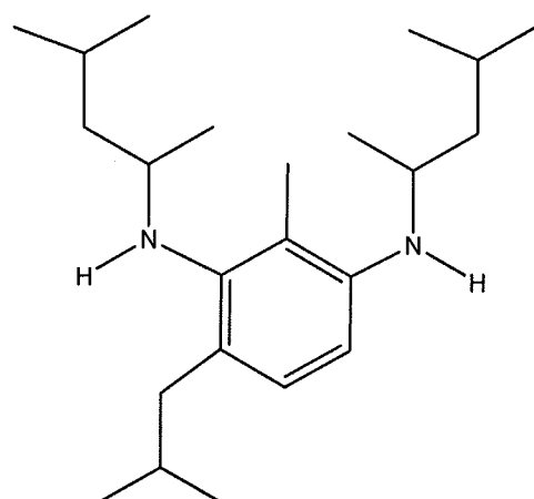
(XXIX);
