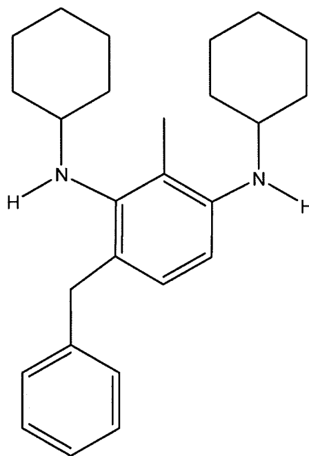
(XXXIV); or
