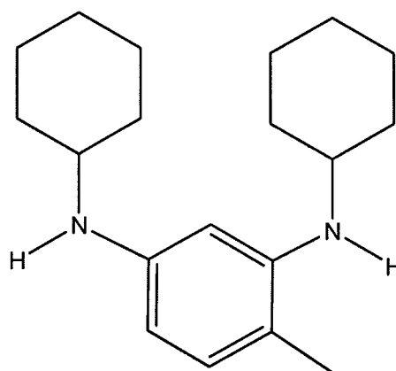
(XXVI);
