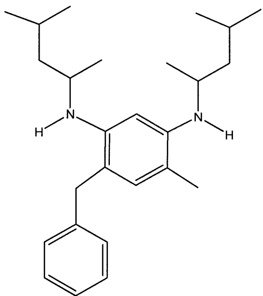
(XXVI);
