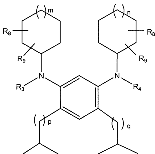
(VIII)
