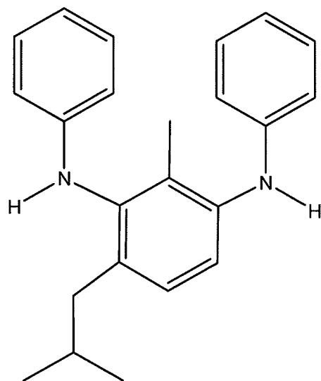
(XXXIV); or
